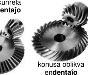
konusa endentaĵo
