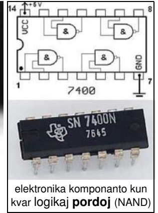
kluzpordeto
