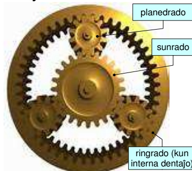
dentrada planedaro
