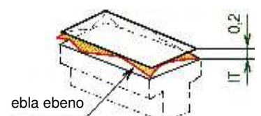
tolereca intervalo de ebena
