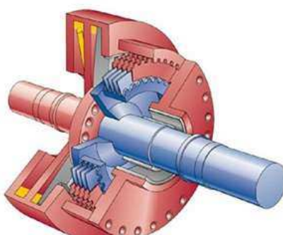
multdiska hidraŭlika kluĉilo
