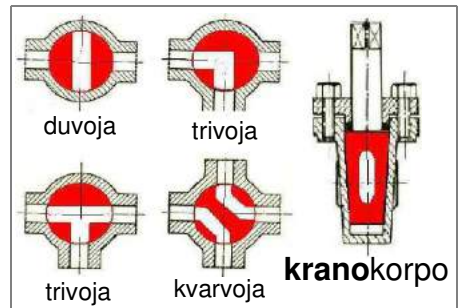
kranko
