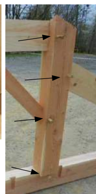
ĉarpentaj keĵloj
