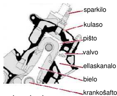
eksplodmotoro
