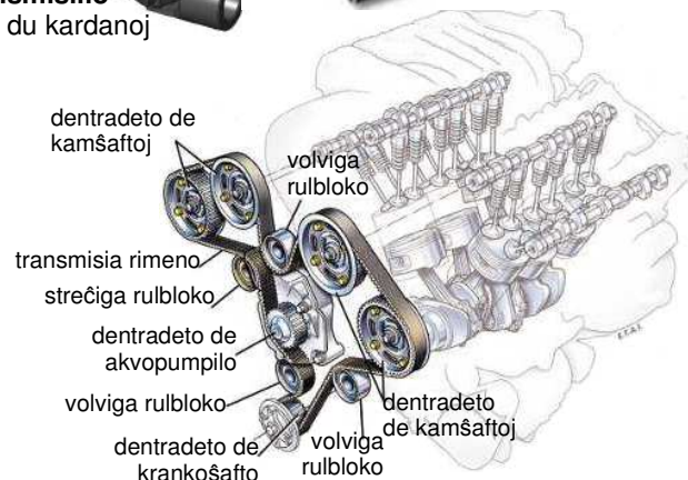
perrimena transmisiilo (motoro V6 24 valvoj)
