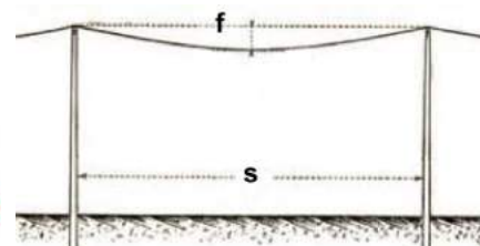
intermasta spano kaj fleksosago
