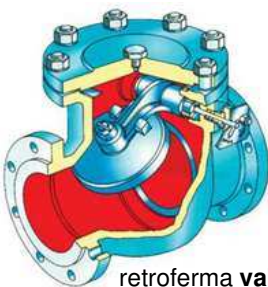
retroferma valvo
