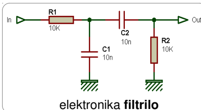
elektronika filtrilo
