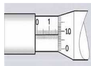
verniero sur mikromezurilo (tie montras valoron de 16,08mm)
