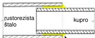
brazajo (tie sur du malsamaj metaloj)
