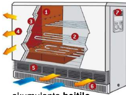
elektra gisa inercia hejtilo
