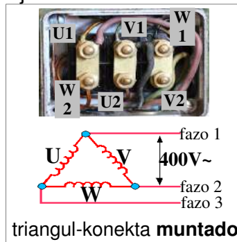
stel-konekta muntado
