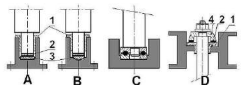
pied-lagro kun glitpeco aŭ glob-lagro
