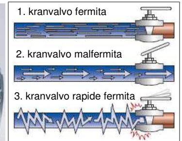
premfrapo kaŭze de kranvalvo
