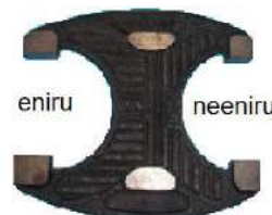
Devomezuro = akcepta flanko Rifuzmezuro = rifuza flanko forka limkalibrilo 30g6
