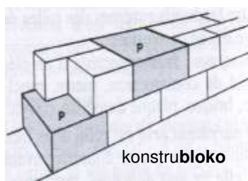
gipsa konstrubloko
