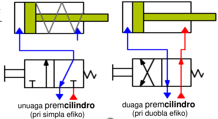
hidraŭlika cilindro
