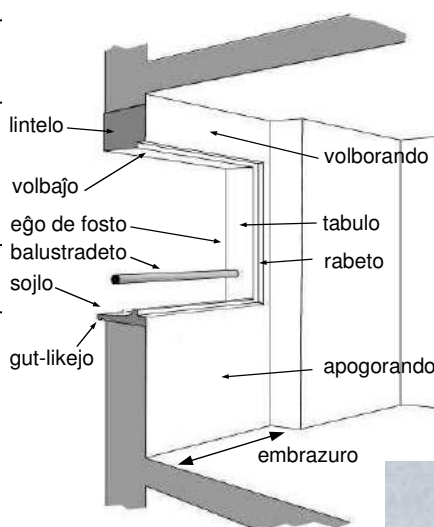
embrasuro de fenestro
