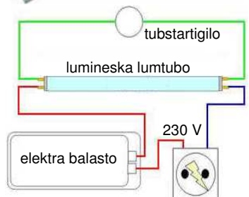
konektoskemo de elektra balasto en tubolumilo
