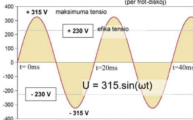
alterna kurento de 230V
