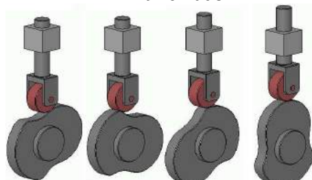
vertikalan movon okazigi per rotacio de kamo
