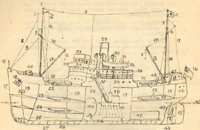
Fig. 2 Kargoŝipo
